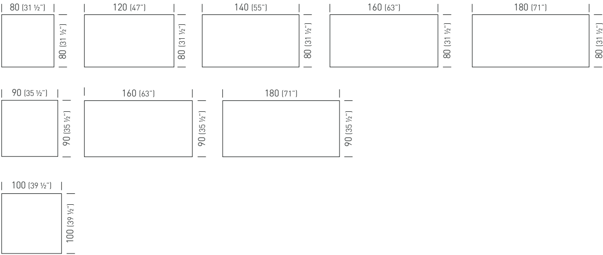
Square section leg Sezione gamba quadrata
