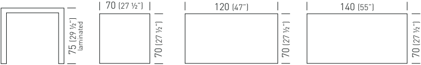
Square section leg Sezione gamba quadrata
